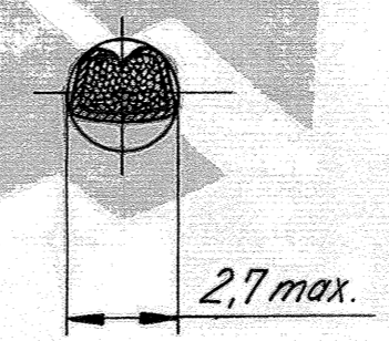
Schnitt C-C
